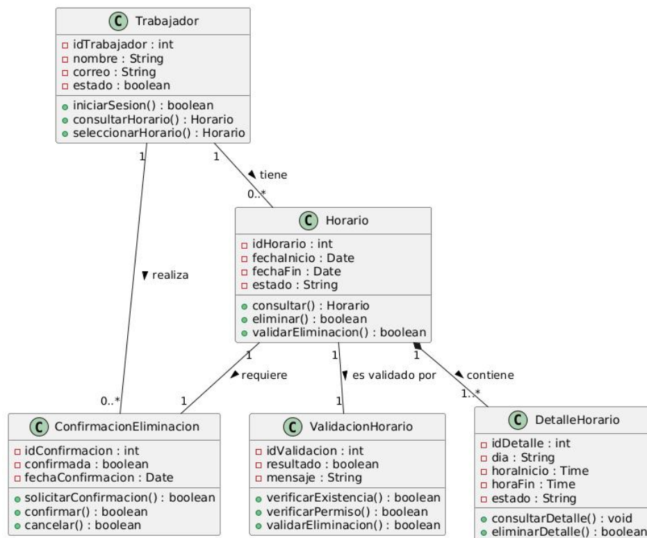
Diagrama de Clases - RF-10 Eliminar Horario
