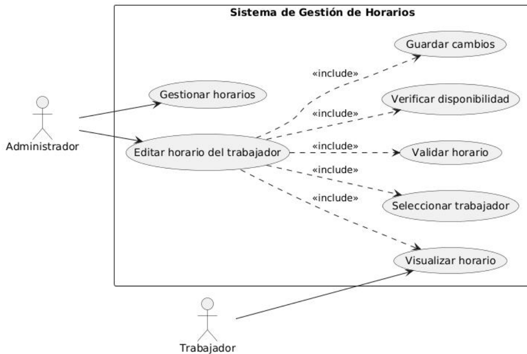
Diagrama de Casos de Uso - RF-11 Editar Horario del Trabajador
