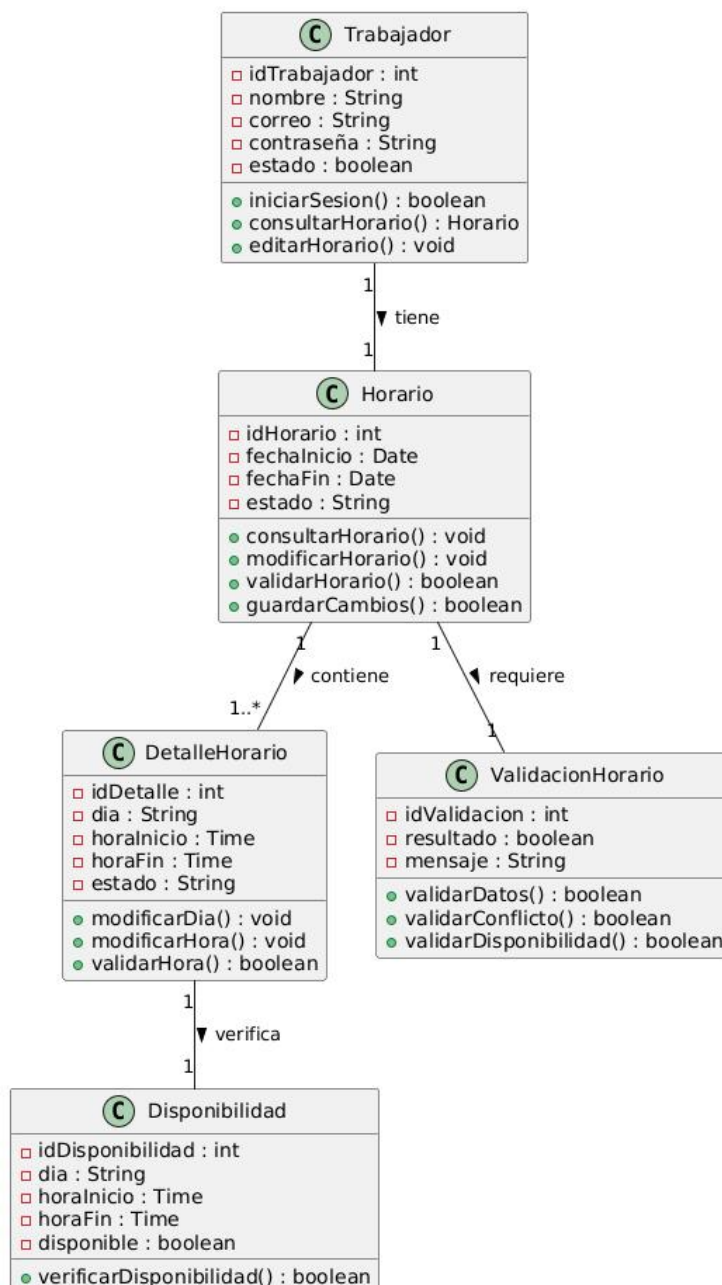
Diagrama de Clases - HU-09 Editar Horario
