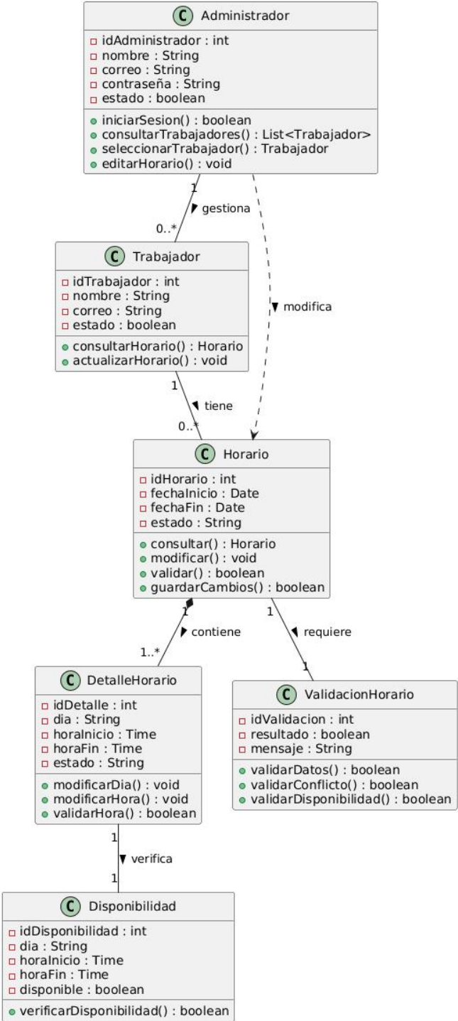
Diagrama de Clases - RF-11 Editar Horario del Trabajador
