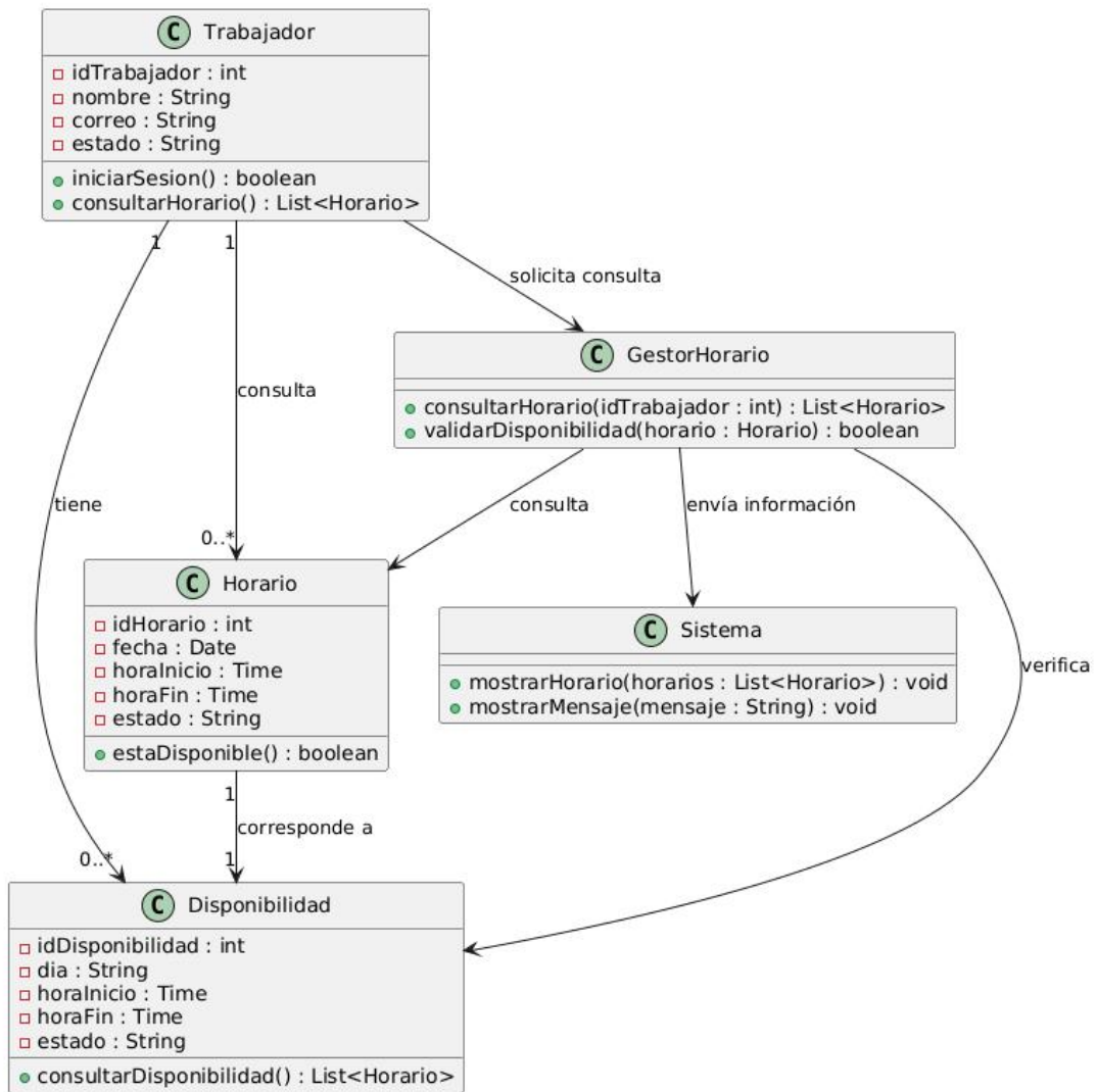
Diagrama de Clases - Visualizar Horario Disponible
