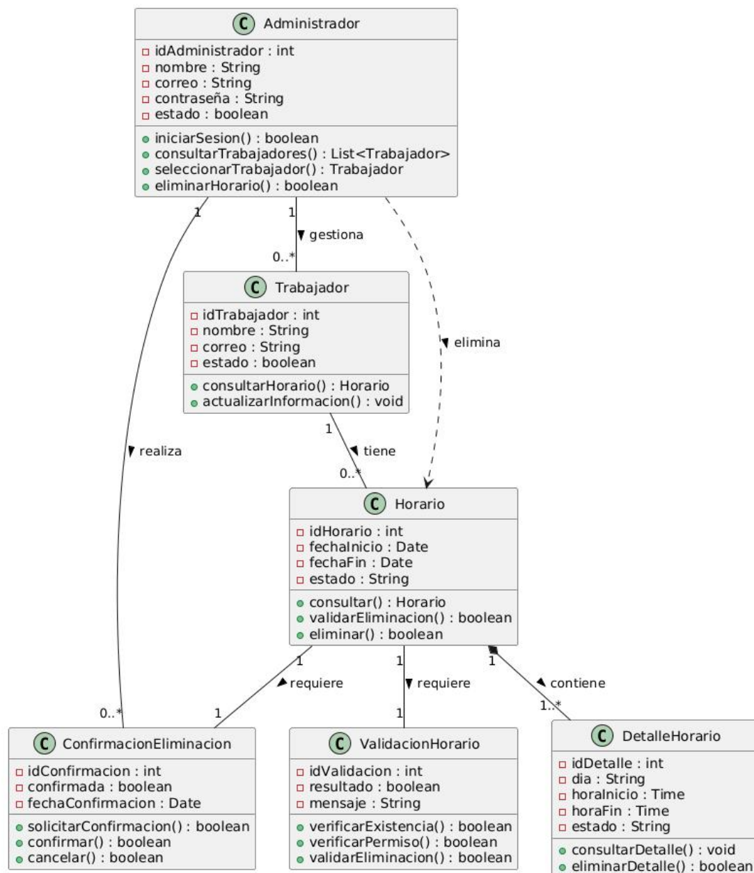
Diagrama de Clases - RF-12 Eliminar Horario del Trabajador
